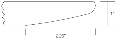
Edge Detail # 38
